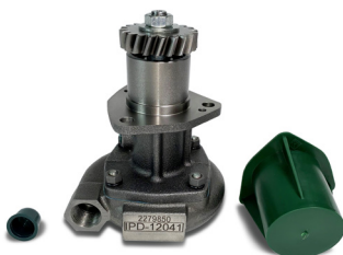
2279850 - G3300 Bomba de agua auxiliar
